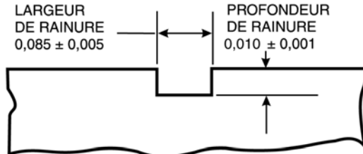
DETAIL D'UNE RAINURE DE VERROUILLAGE
