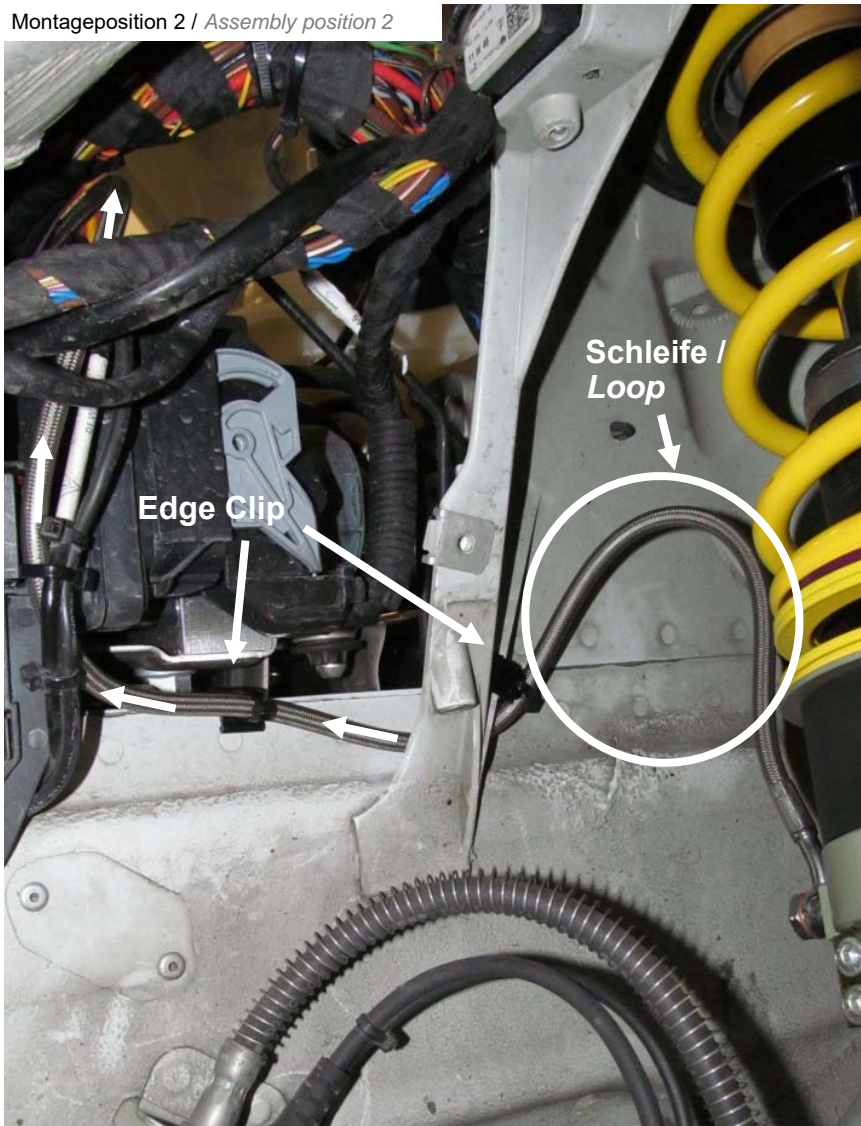
Edge Clips
