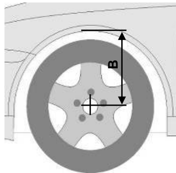
Abstandsmaß B - Radmitte - Kotflügelunterkante
