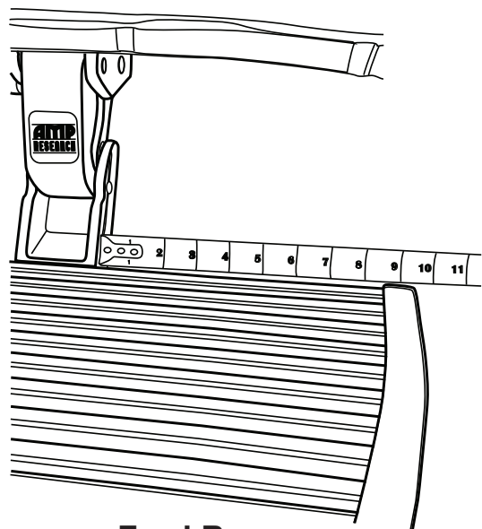
4 Ford Bronco
